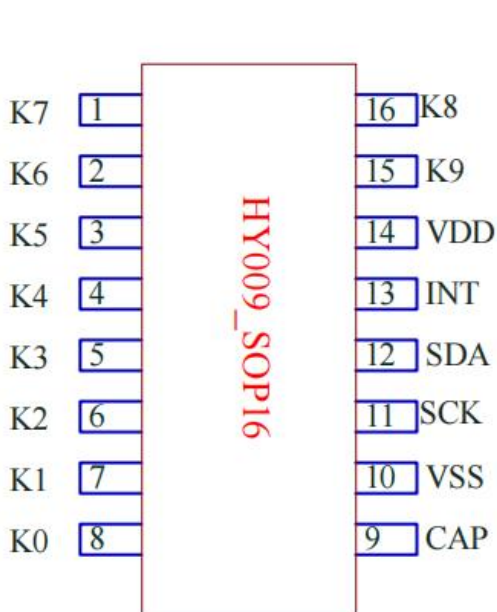
Sop16
