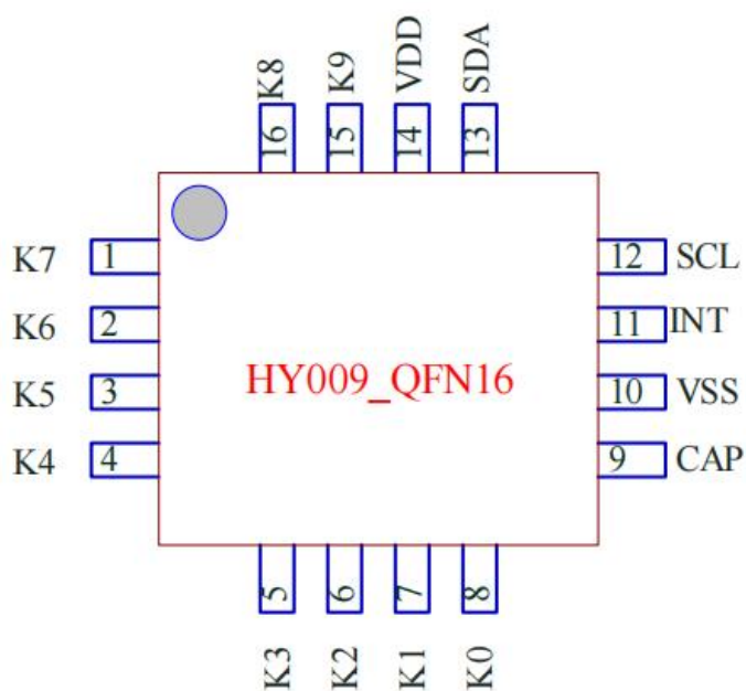
QFN16
