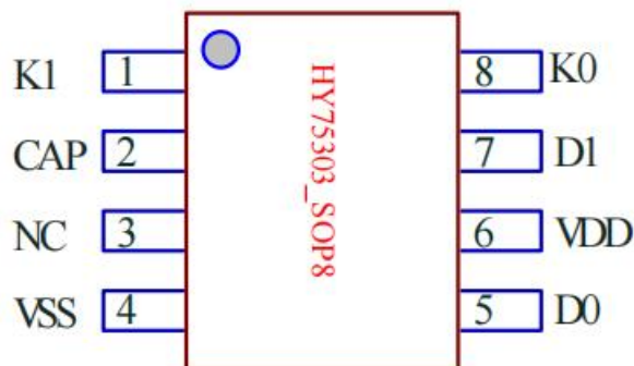
SOP8
